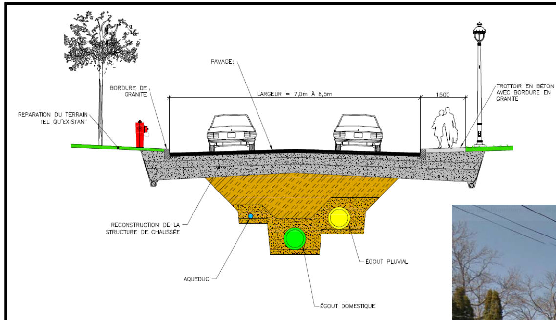
Coupe type chaussée
